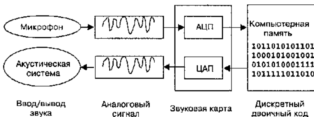
Рис. 5.3. Преобразование звука при вводе и выводе
