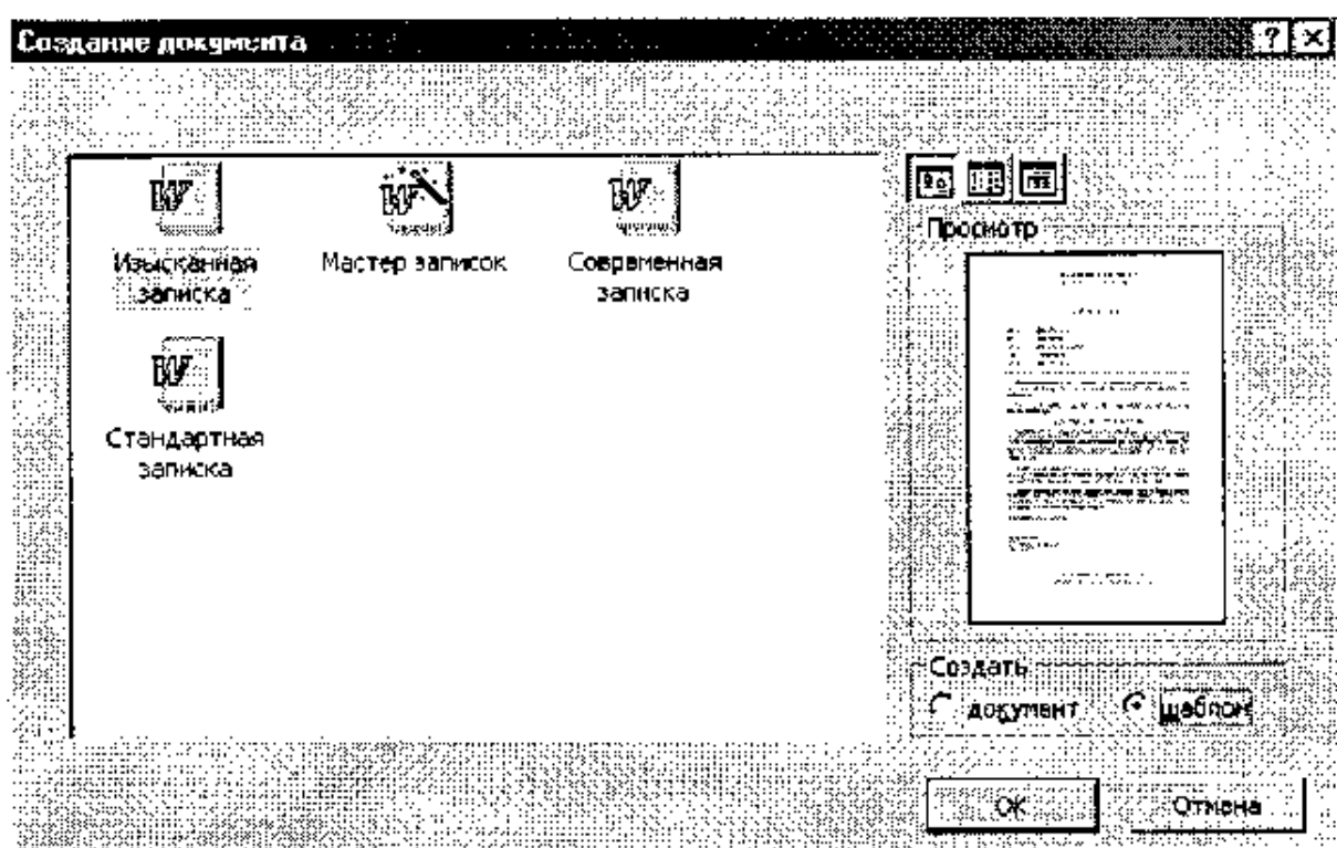
Рис. 3.3. Шаблоны документов
